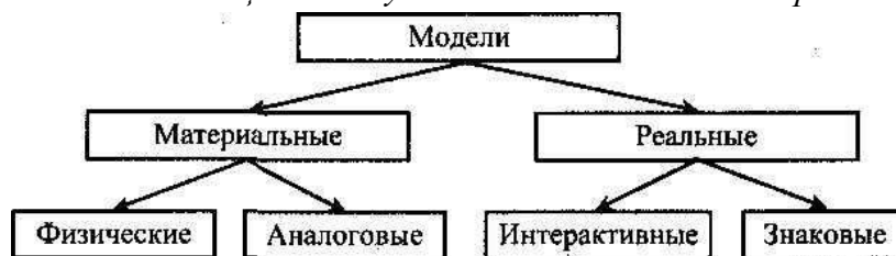
Рис. 1. Классификация моделей
