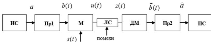
Рис. 1.2. Упрощённая структура системы связи
