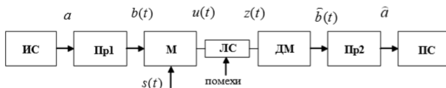
Рис. 1.2. Упрощенная структура системы связи
