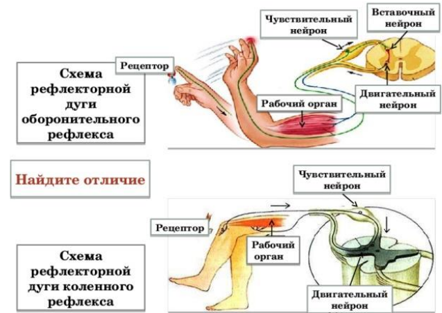
Рисунок 1 – Схема простой и сложной рефлекторной дуги
